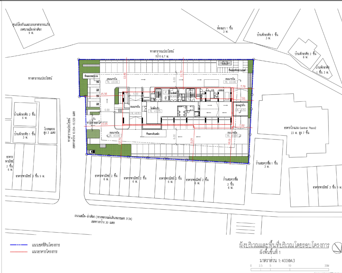
ผังบริเวณโครงการก่อนเปลี่ยนแปลง
