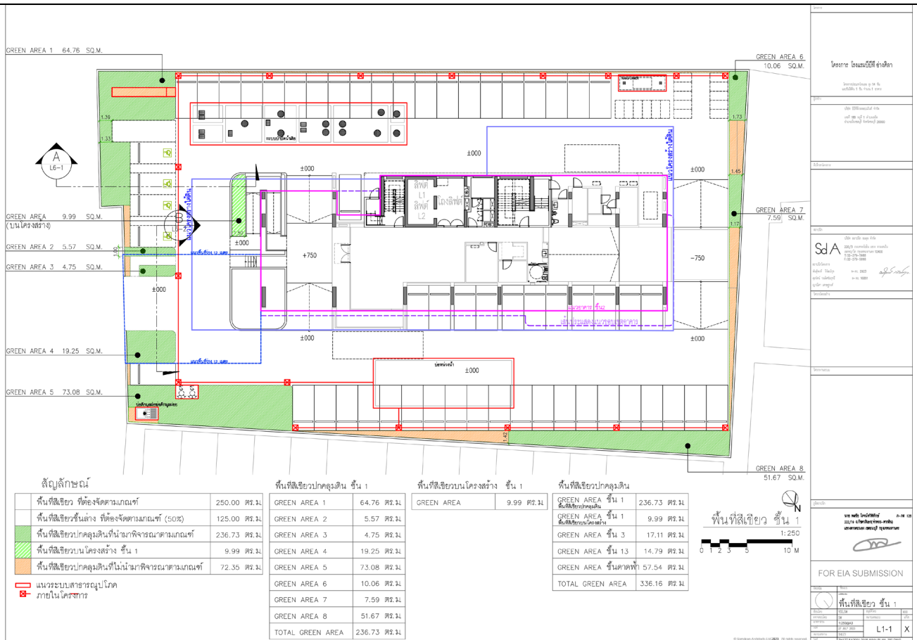
ผังพื้นที่สีเขียวบริเวณชั้น 1 ก่อนเปลี่ยนแปลง
